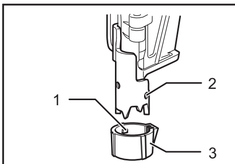
► 1. Protrusion 2. Hole 3. Nose adapter
