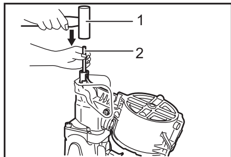
► 1. Martillo 2. Varilla pequeña
