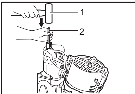
► 1. Hammer 2. Small rod
