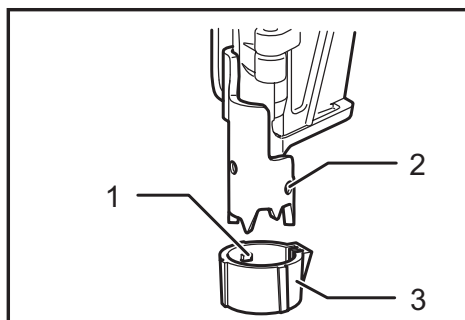
► 1. Protuberancia 2. Orificio 3. Adaptador de nariz
