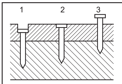
► 1. Profundidad excesiva 2. Al ras 3. Superficialidad excesiva
